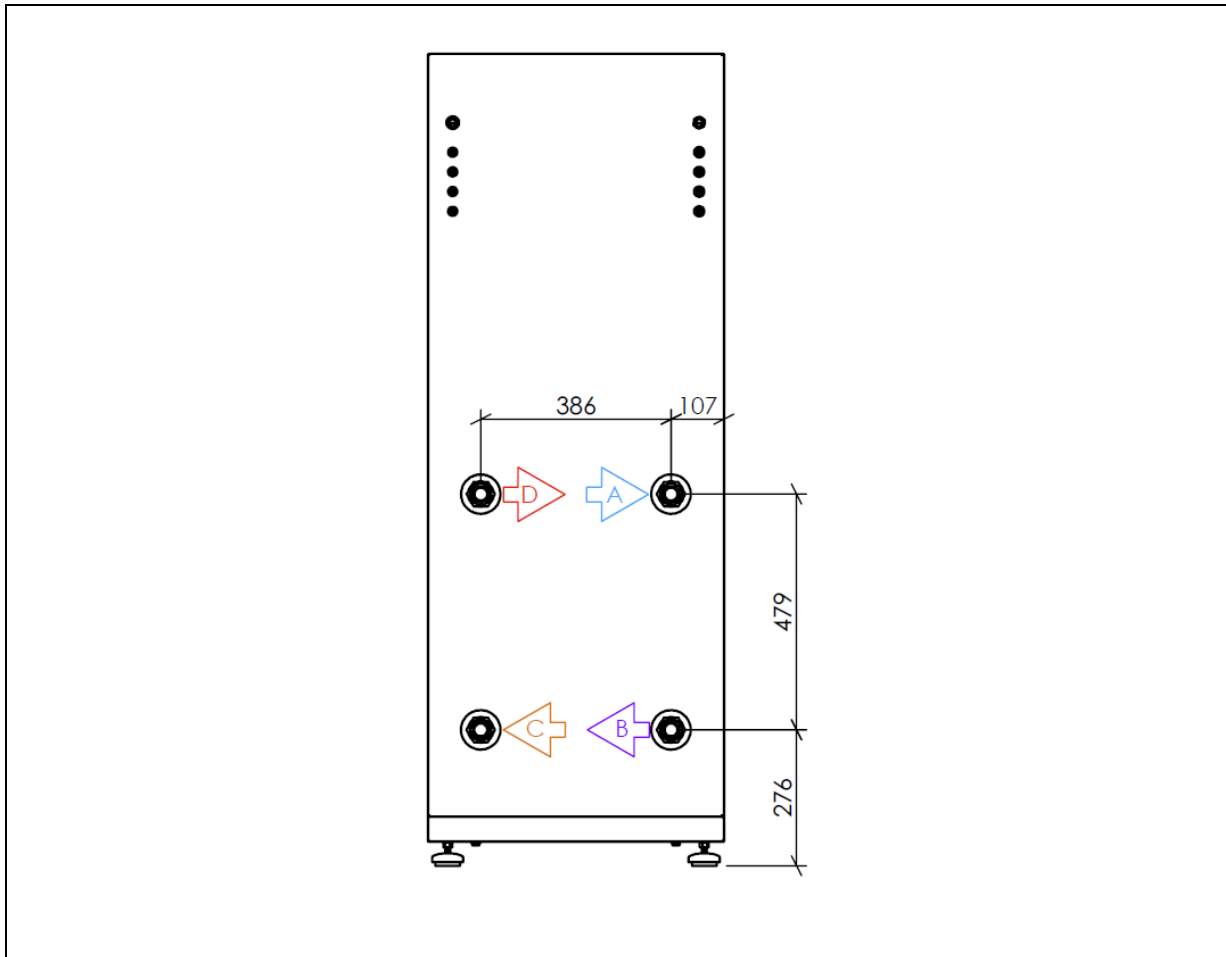
Rys. 9: Tylna strona obudowy pompy ciepła EUROS GEO.
