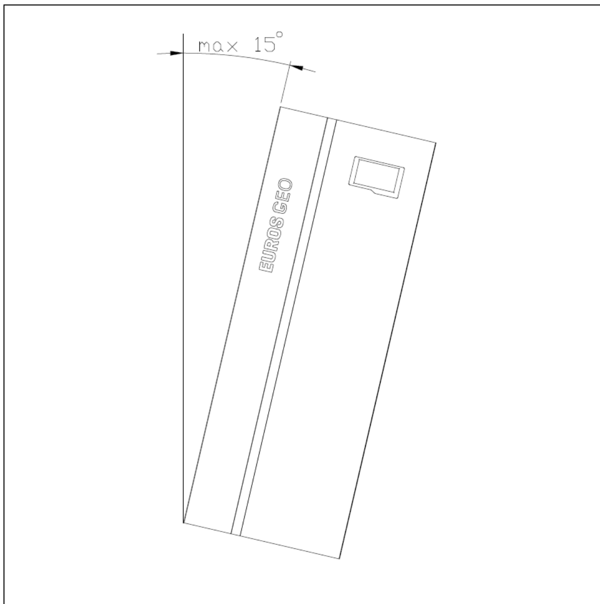
Rys. 7: Maksymalny przechył pompy ciepła EUROS GEO w czasie transportu.
