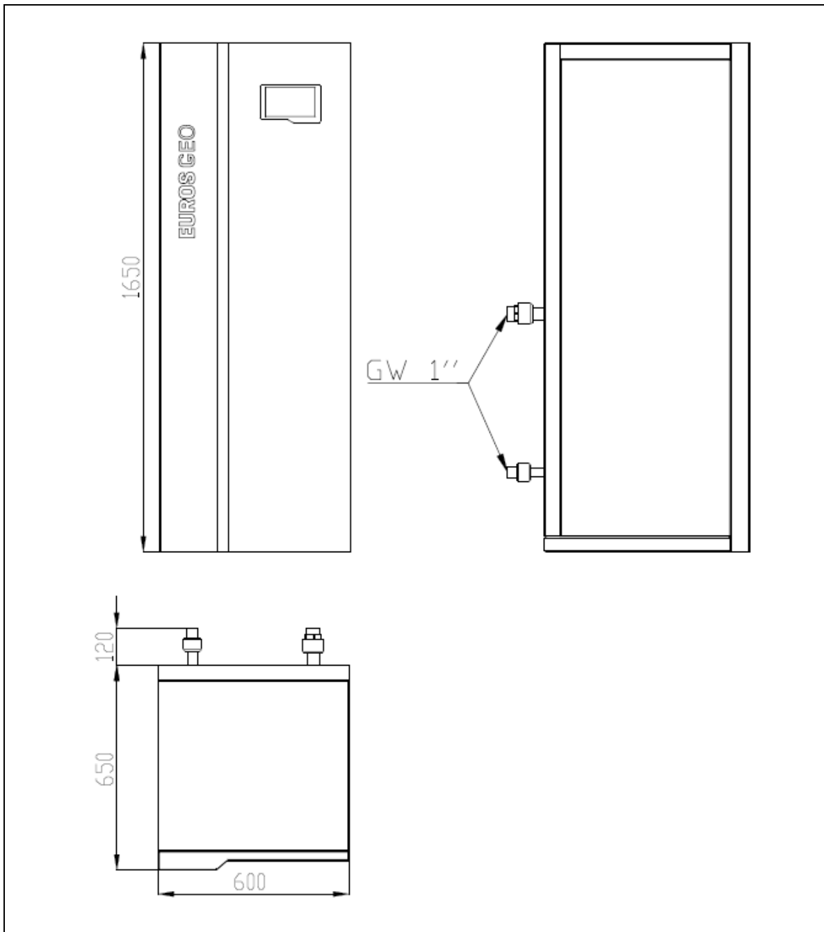
Rys. 6: Gabaryty jednostki wewnętrznej pompy ciepła EUROS GEO
