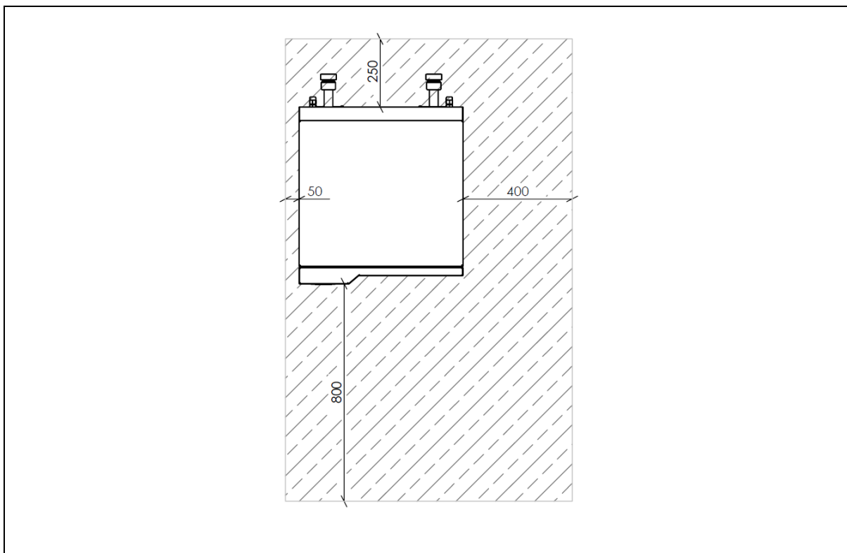
Rys. 8: Ograniczenia dotyczące miejsca ustawienia pompy ciepła EURO S GEO z wyjątkiem pracy w kaskadzie.
