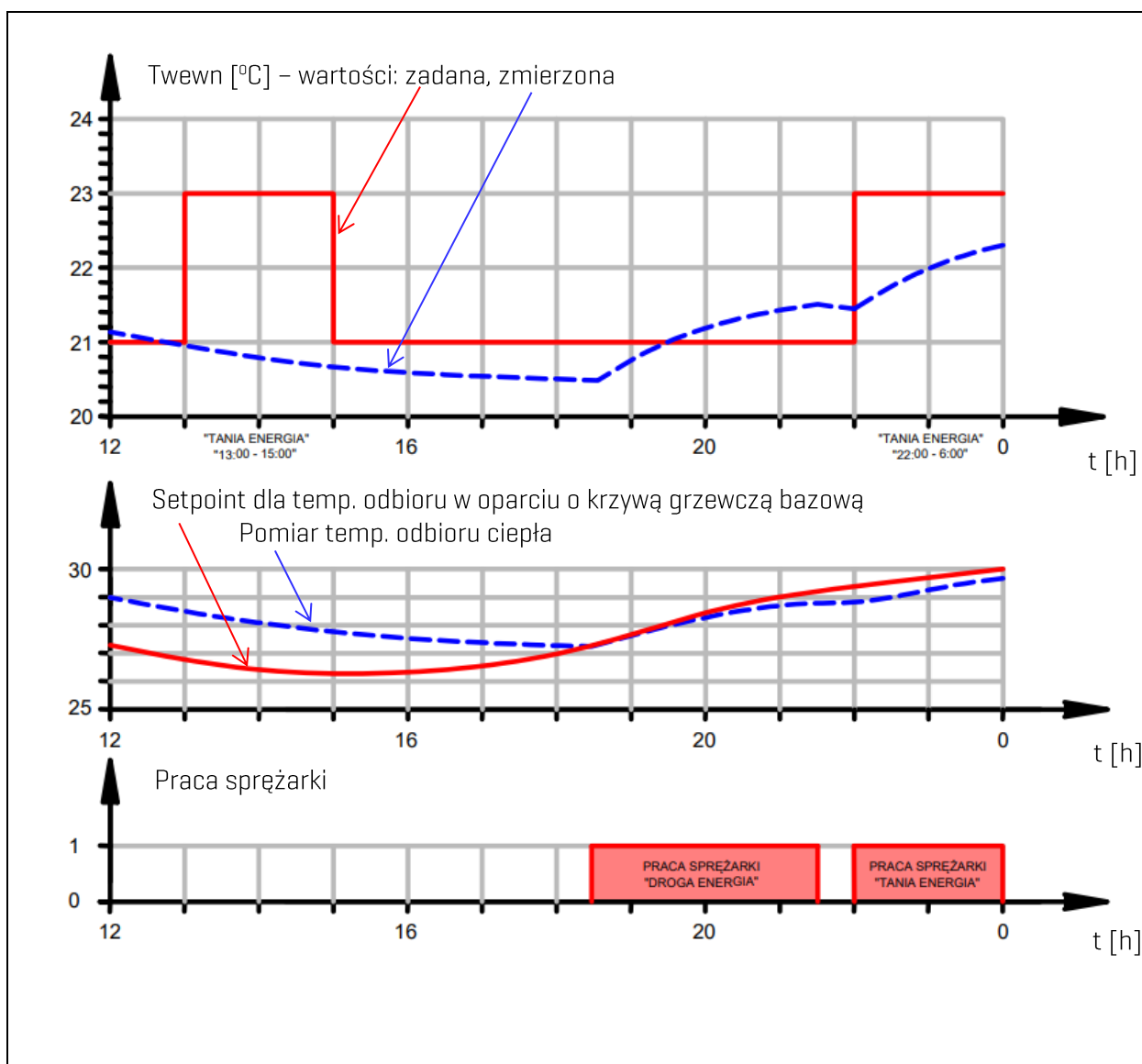
Rys. 14: Automatyczna zmiana temperatury zadanej w trybie ECO bez wykorzystania mechanizmu REG+.
